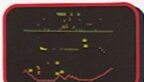
Planetoid
